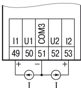
Рисунок 6 – Подключение активного датчика с выходом типа «Ток 4...20 мА»
